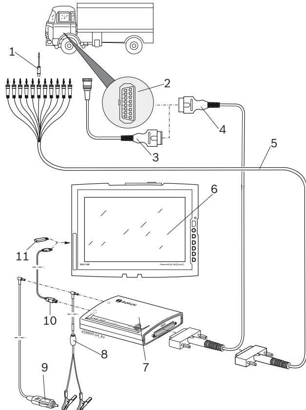
Abb. 3: Kapcsolási rajz KTS Truck
