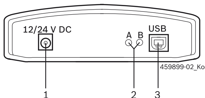
Abb. 2: Barrette de connexion
