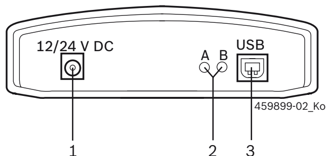
Abb. 2: Pannello di collegamento
