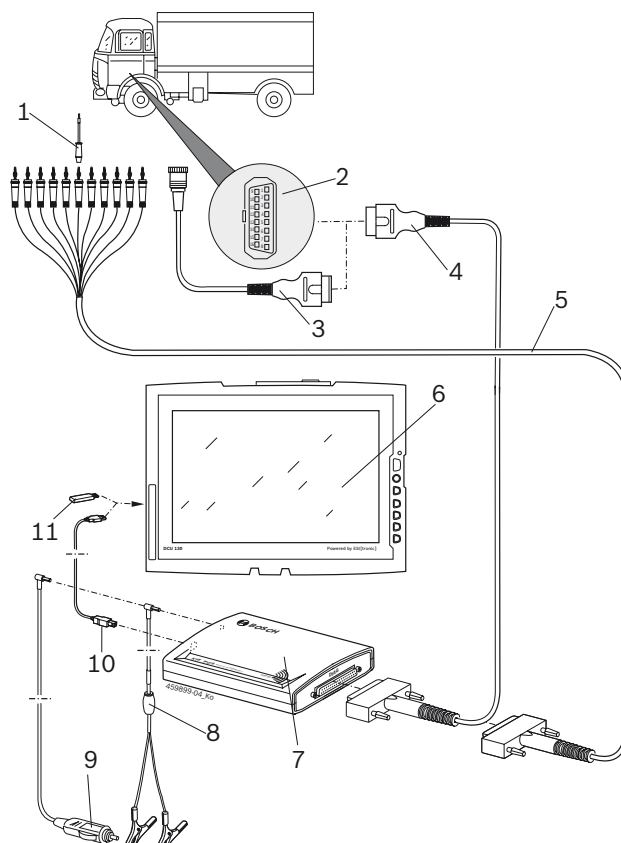
Abb. 3: Schemă de conexiuni KTS Truck
