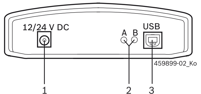
Abb. 2: Bară de conexiune
