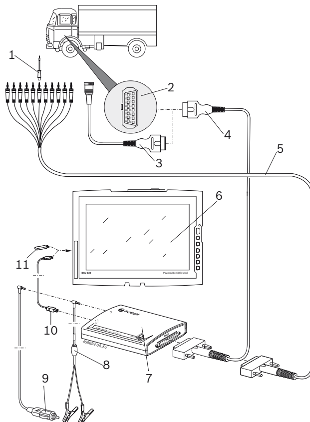
Abb. 3: Anschlussplan KTS Truck
